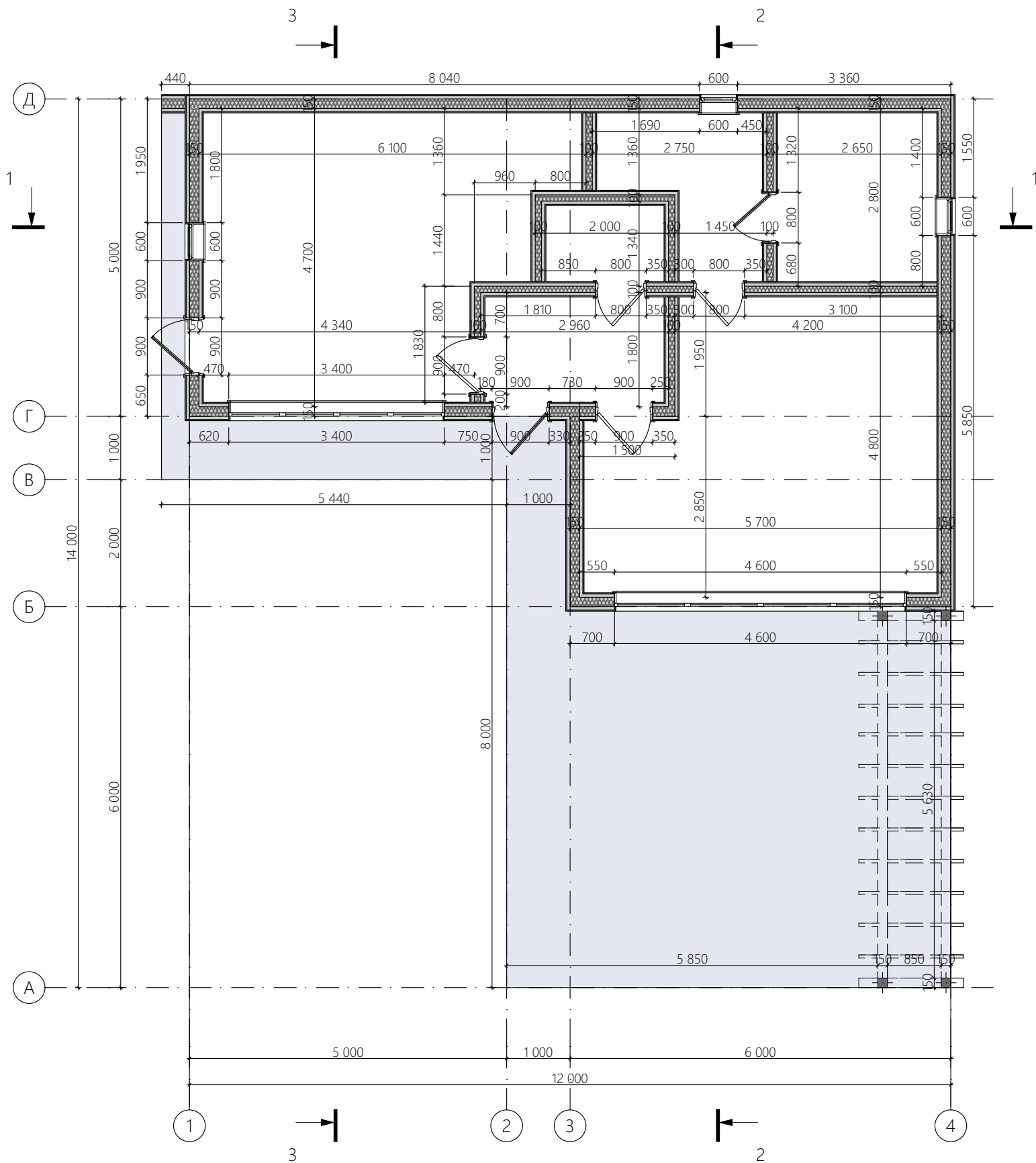
Размерный план
